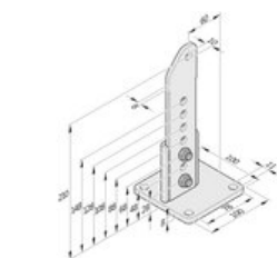
Toripostenbeschlag 60/210 L
