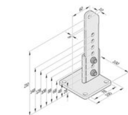
Toripostenbeschlag 60/210 R
