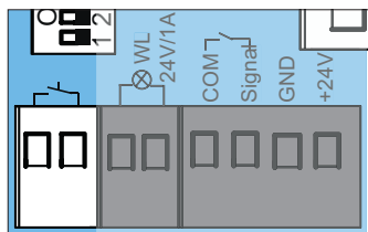
Рис. Разъем для кнопки
