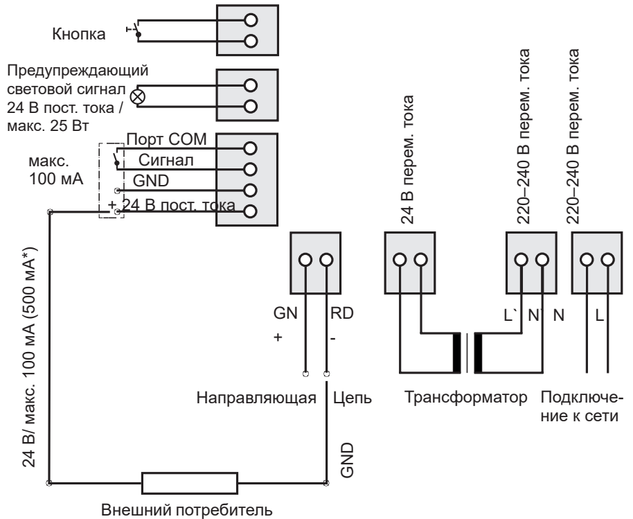
Рис. Схема подключения Потолочный блок управления
