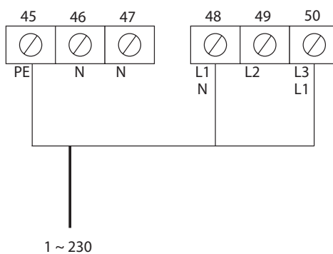
Raccordement secteur
